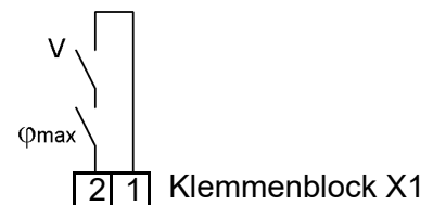
Klemmenbeschaltung 1/2 am Klemmenblock X1 für den Anschluss der Sicherheitskette
