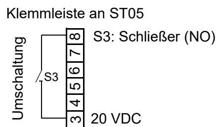
Klemmenbeschriftung 3/8 an der Erweiterungsplatine zur Umschaltung zwischen Zuluftbefeuchtung (S3 offen) und Abluftkühlung (S3 geschlossen) bei Kombinationsanlagen unter Nutzung des Digitaleingangs
