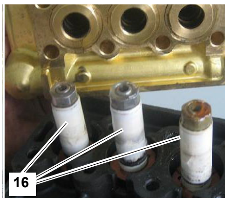
Keramikkolben
