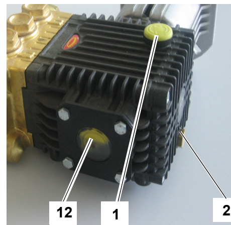
Einfüllöffnung, Schauglas und Entleerungsschraube
