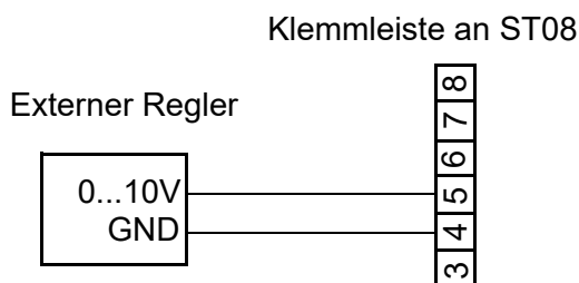
Klemmenbeschriftung 4/5 an der Hauptplatine (Klemmleiste an ST08) für den Anschluss eines externen Steuersignals 0...10V
