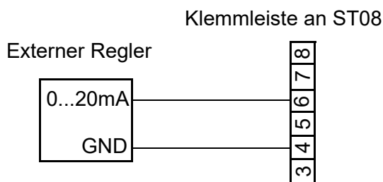
Klemmenbeschriftung 4/6 an der Hauptplatine (Klemmleiste an ST08) für den Anschluss eines externen Steuersignals 0...20mA
