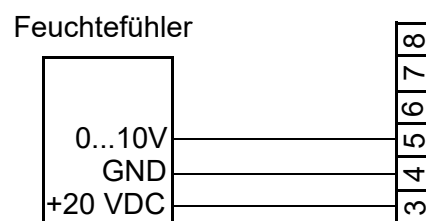
Klemmenbeschaltung 3/4/5 auf der Hauptplatine (Klemmleiste an ST08) für den Anschluss eines aktiven Feuchtefühlers 0...10 V
